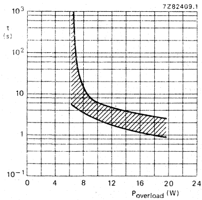
Fig. 4 NFR25; R > 100 .
